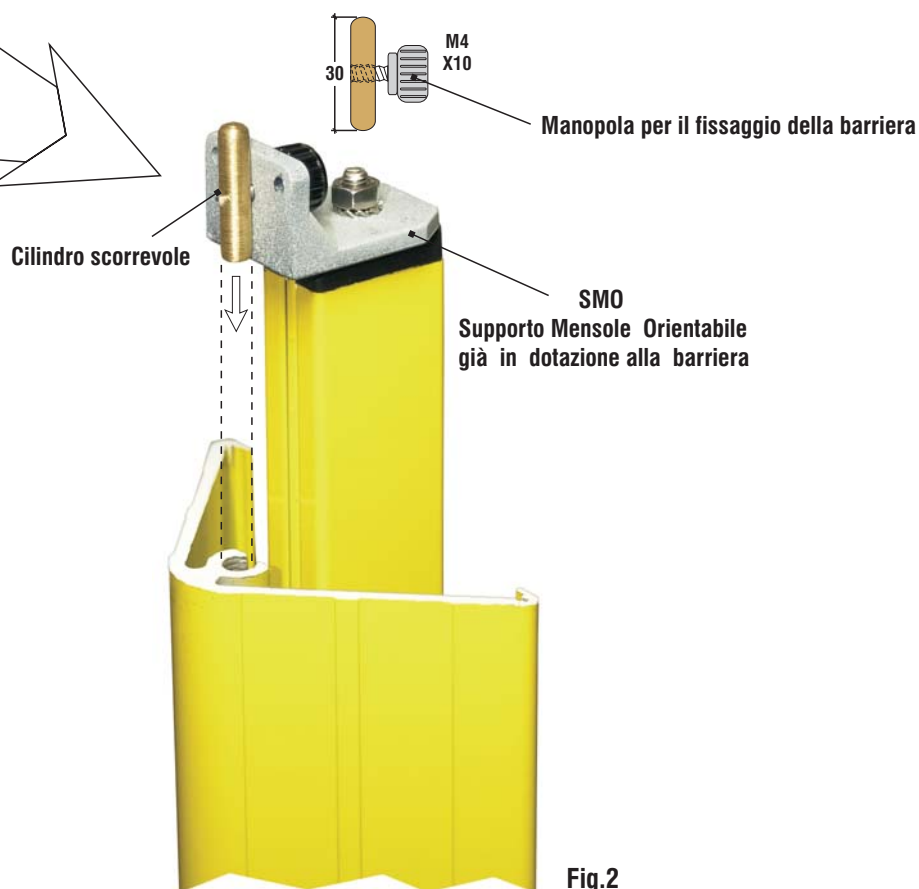
PARTICOLARE DELLA MENSOLA SUPERIORE
